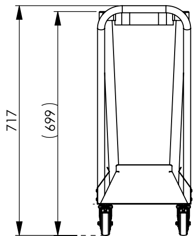
Jäätmenõuga (lisana)/ With Waste Bin (as extra)
